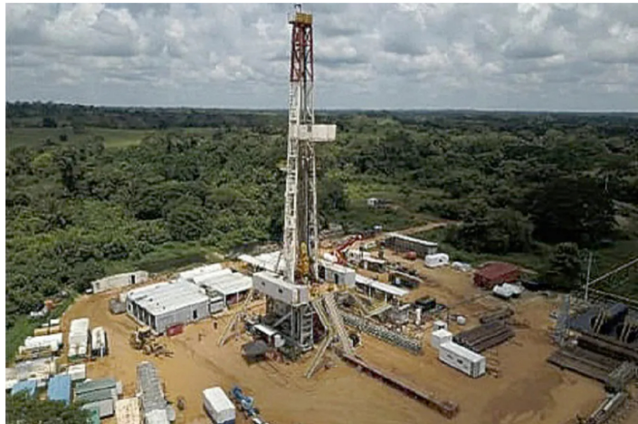
Campo de gas Arrecife, municipio Pueblo Nuevo, Córdoba. Hocol ratifica el compromiso de mantener los esfuerzos exploratorios en las cuencas del Caribe colombiano para el hallazgo de nuevas reservas de gas y la aceleración de su puesta en producción.
