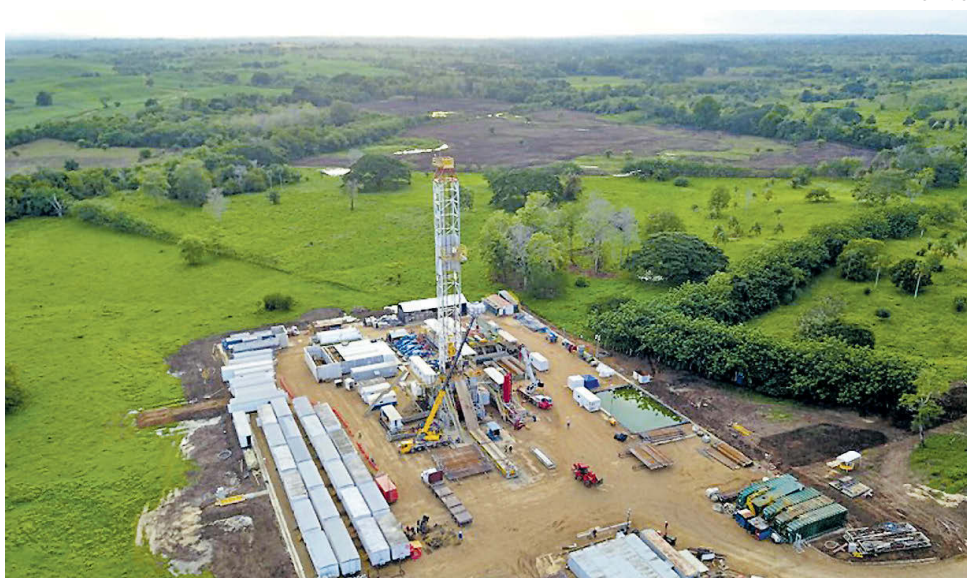
Pozo Aguas Vivas de Canacol ubicado en Sahagún, Córdoba.
